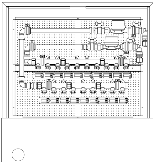
Kytkentä alajakoisesti 9+10 lähtöä
