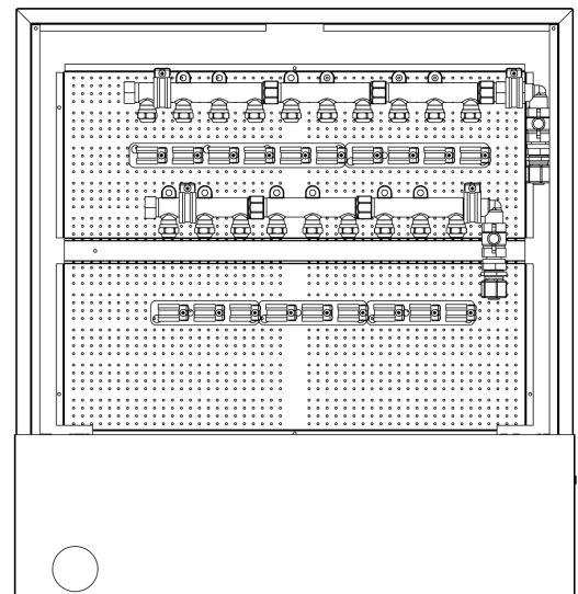
Kytkentä ilman vesimittareita 9+10 lähtöä
