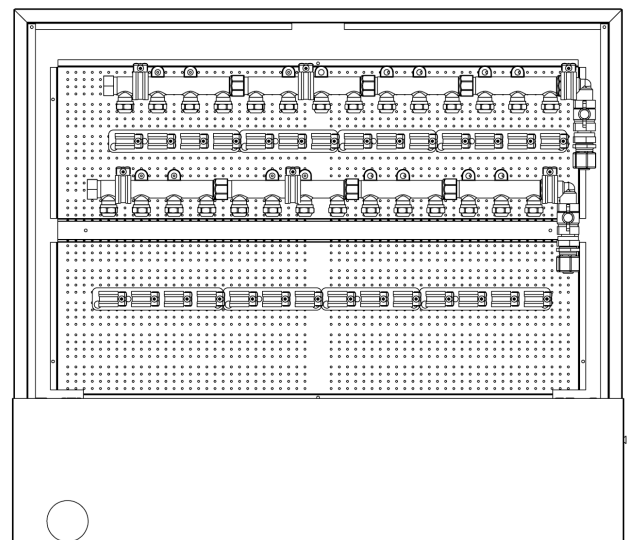
Kytkentä ilman vesimittareita 14+14 lähtöä
