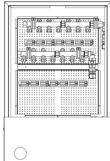
Kytkentä ilman vesimittareita 7+7 lähtöä
