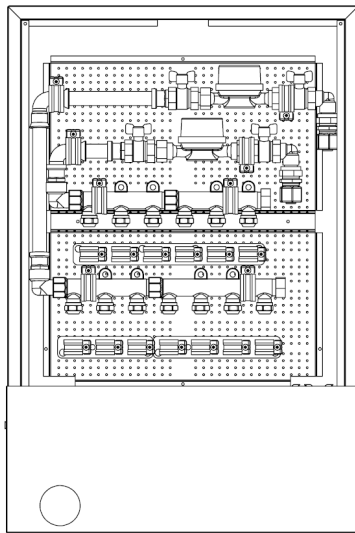
Kytkentä alajakoisesti 6+7 lähtöä
