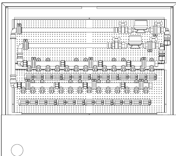
Kytkentä alajakoisesti 14+14 lähtöä
